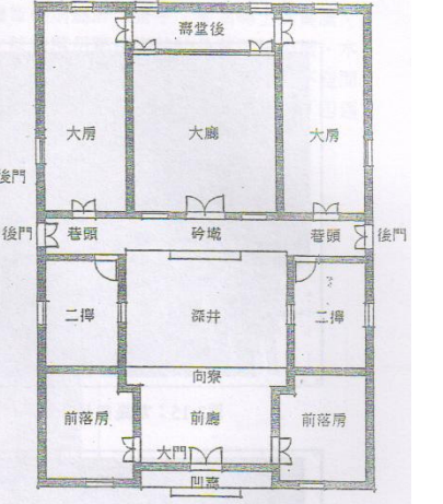
圖2-19：三蓋廊民宅平面佈局(作者繪)
