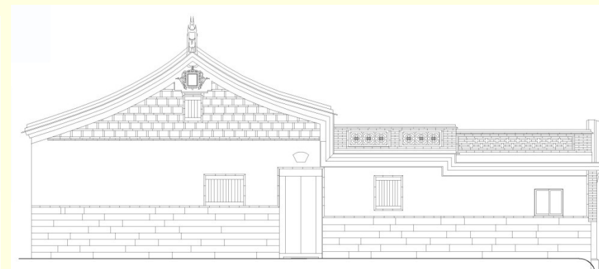
北向立面圖
