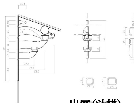
出展(斗拱) 大樣圖
