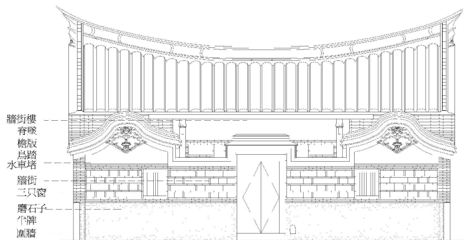
正立面
