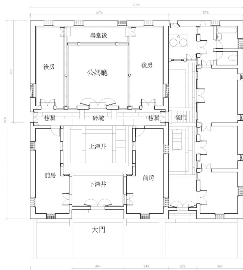
平面圖
