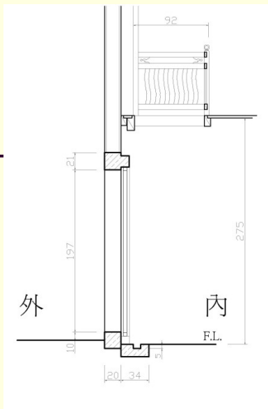
半樓扶手大樣圖
