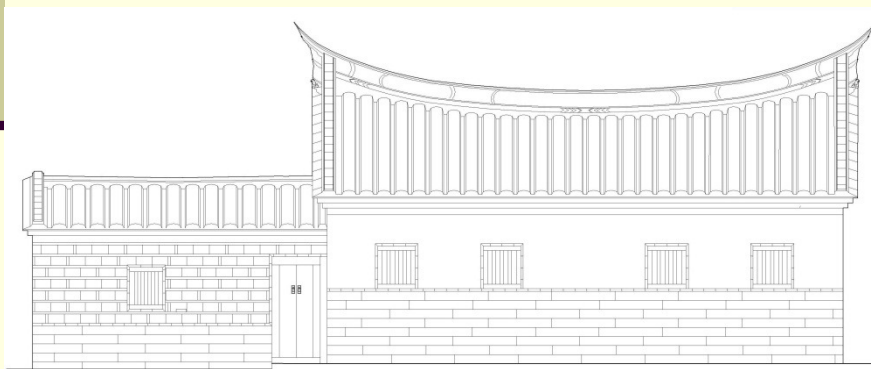
東向立面圖
