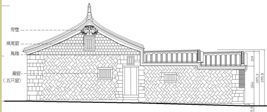
側立面圖
