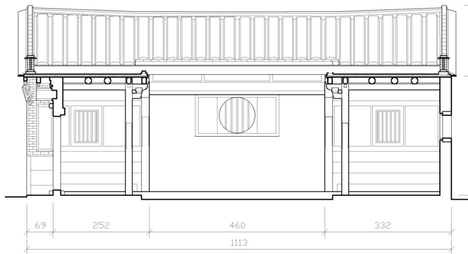
入口過水及深井剖面圖
