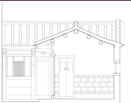
護龍橫剖面圖
