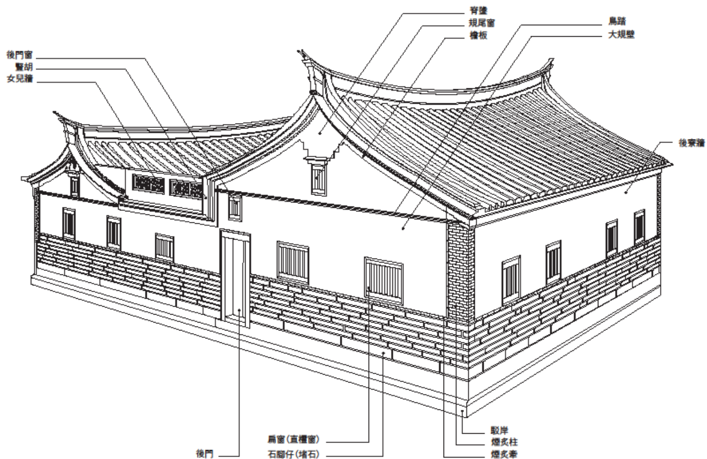
側立面構件說明圖
