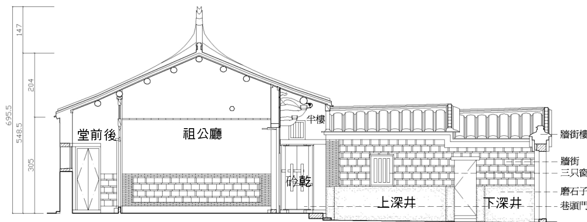
縱剖面圖
