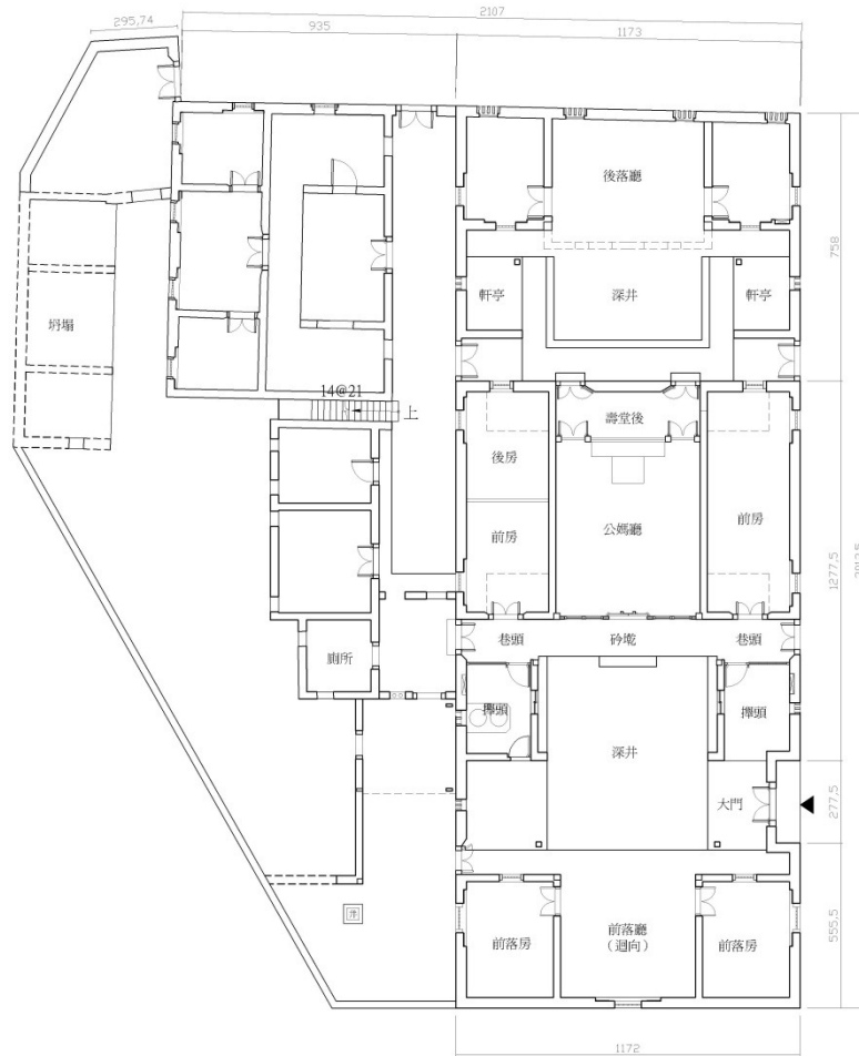
平面圖
