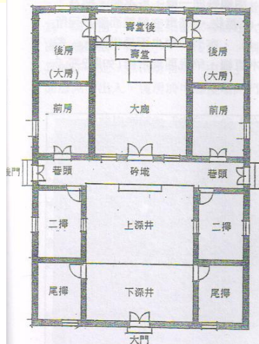
圖2-5：一落四擡頭民宅平面佈局(作者繪)
