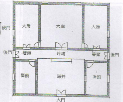
圖2-4：一落兩擡頭民宅平面佈局(作者繪)
