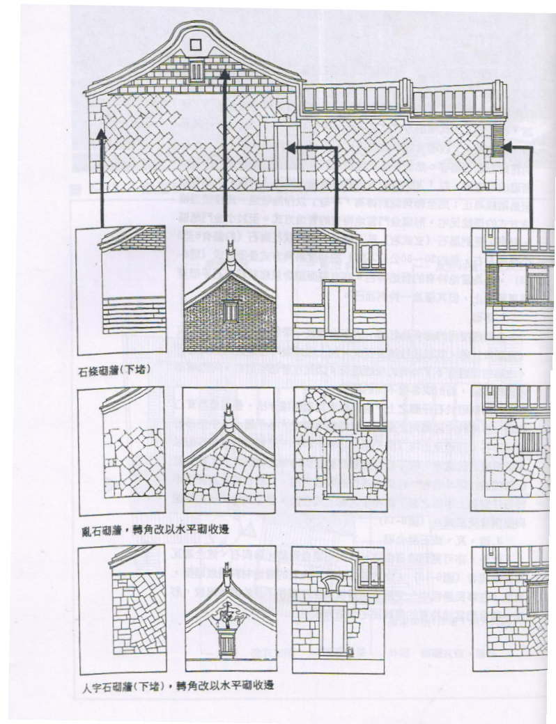
圖：石砌壁體構造類型比對照圖 資料來源:米復國，1994年，《金門與澎湖地區傳統聚落與民宅之調查研究》，行政院文化建設委員會。
