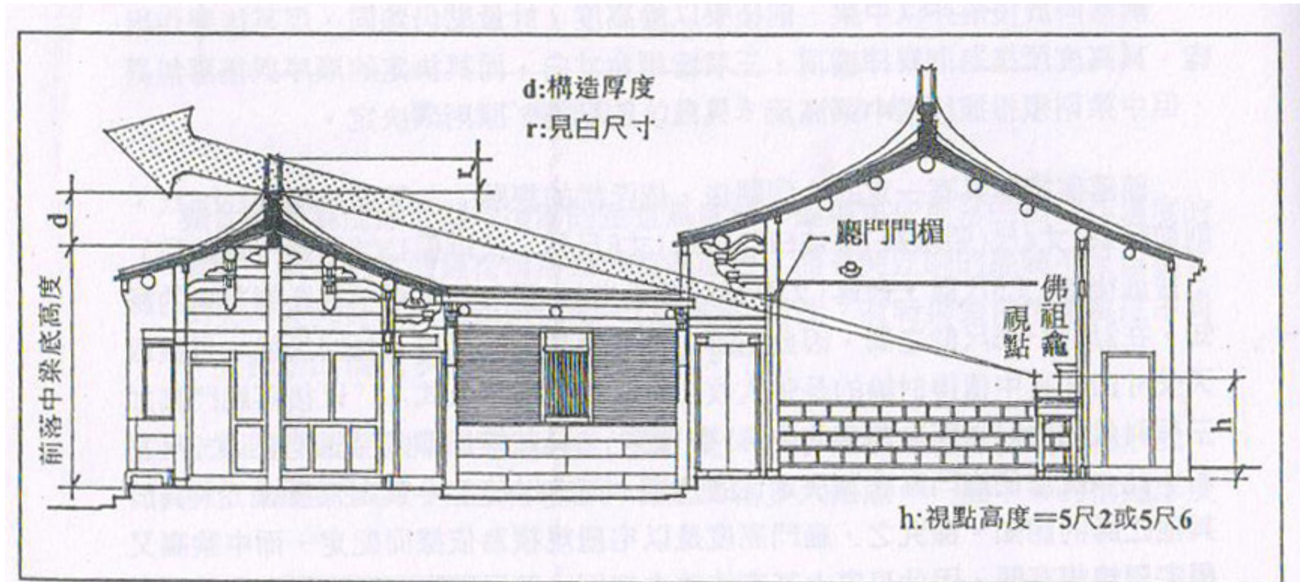
「見白」禁忌/原則——前落高度的定法(作者繪)
