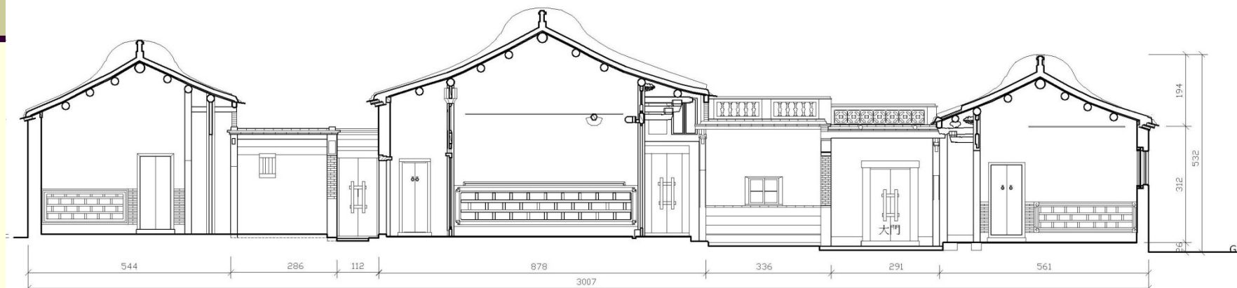
縱剖面圖
