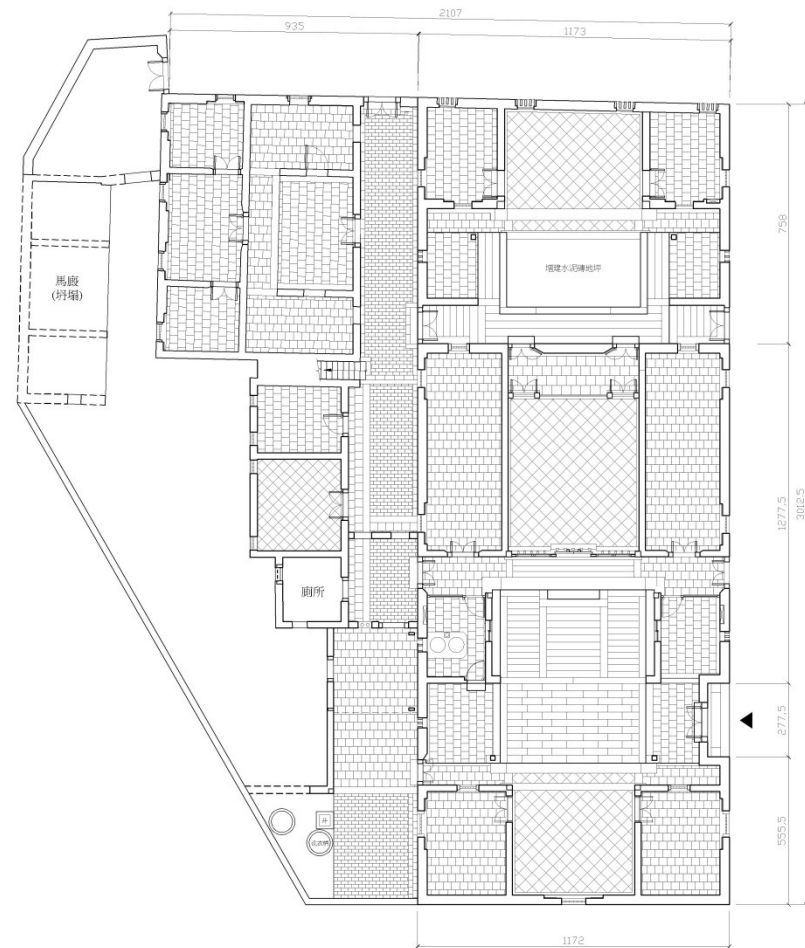
鋪面配置圖
