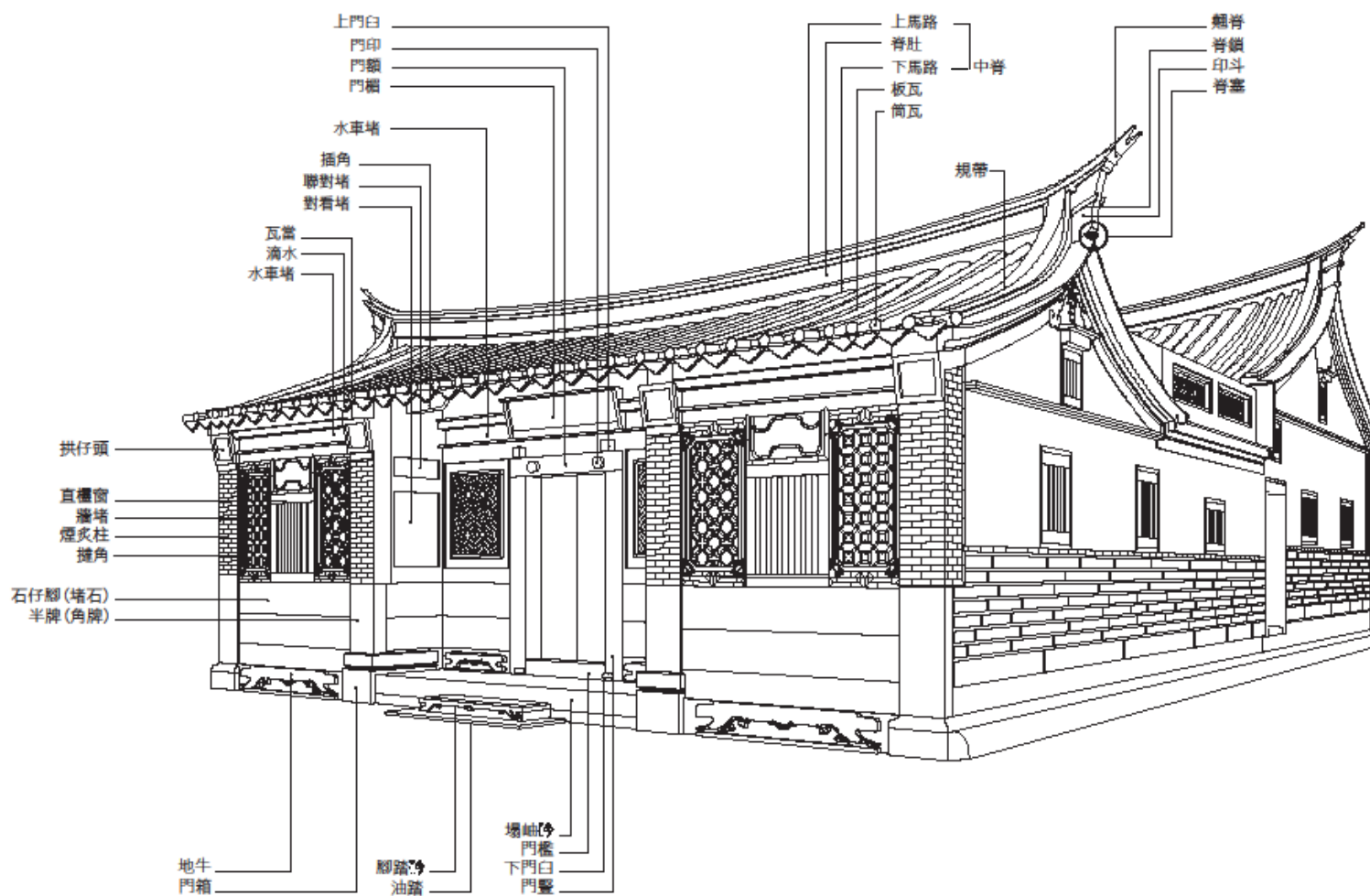
正立面構件說明圖
