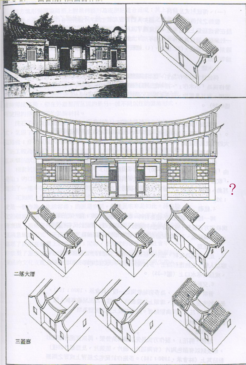
圖：四合院入口凹壽作法
