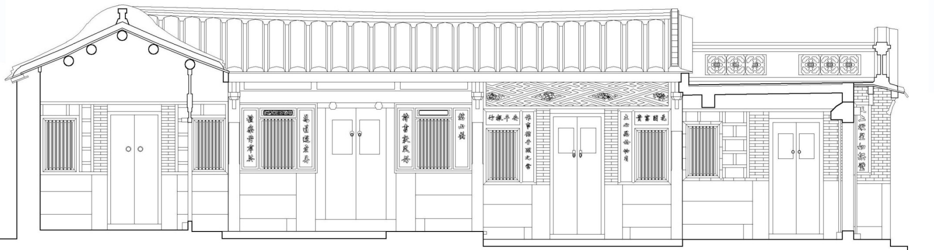
護龍長向剖面圖
