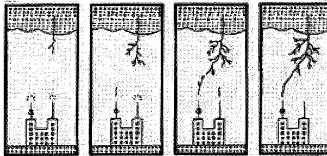
NOVA 提前放電避雷針工作原理
