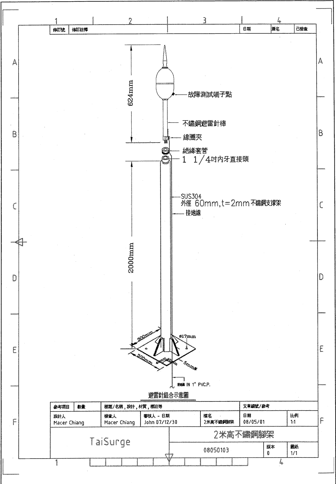
避雷針安裝示意工程圖
