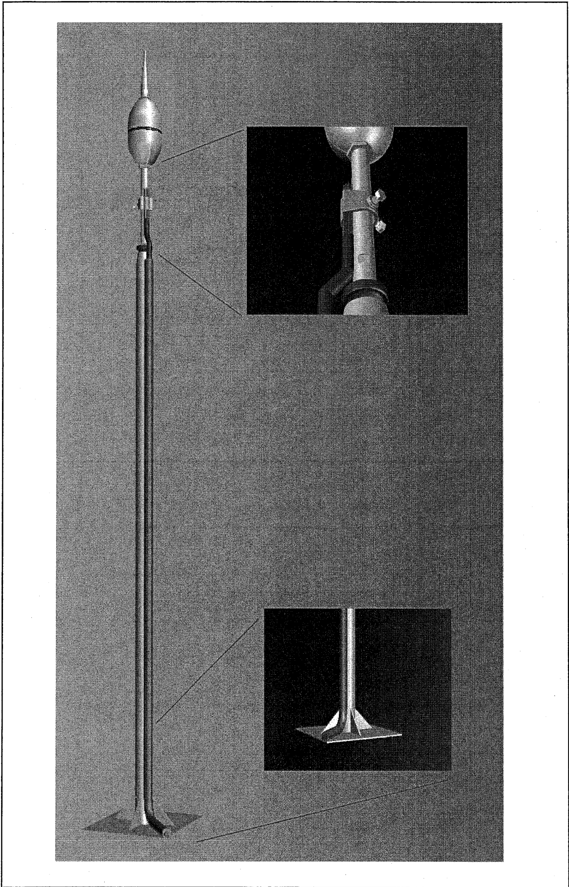
避雷針安裝示意立體圖
