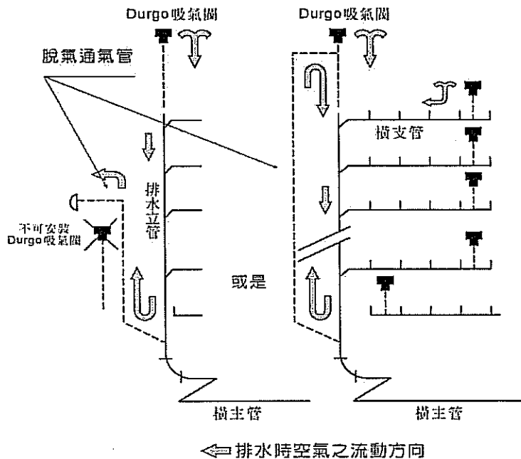
圖 3-10 因排水橫主管 2 公尺內曲折、橫主管管尺寸無法加大而設置逃氣通氣管的排水通氣路徑示意圖
