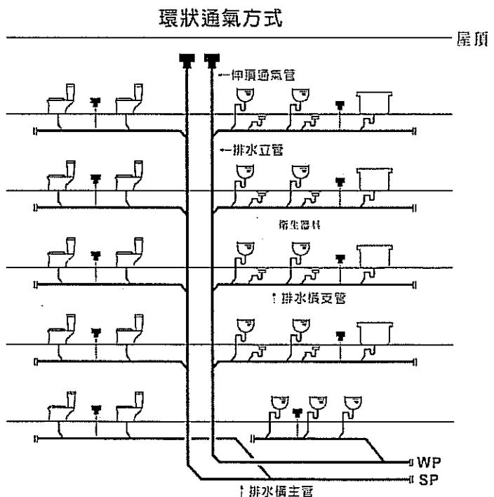
圖 3-6 環狀通氣方式系統使用 Durgo 吸氣閥圖例
