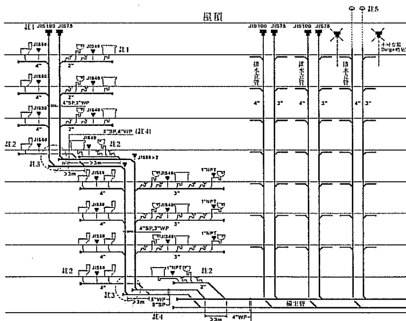
圖 3-2 Durgo 吸氣閥運用於排水立管設有 offset 及橫主管設有三支以上立管群之圖例 (Durgo 編號 AI, BI 吸氣閥之使用例)
