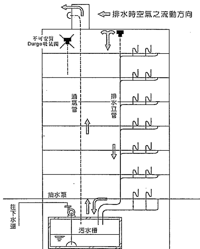
圖 3-8 當排水進入污水槽時對流空氣經由通氣管逃逸的通氣路徑示意圖
