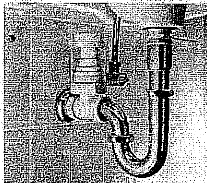
圖 3-15 廚房流理台及浴室洗臉盆排水裝設 1" NPT Durgo 吸氣閥示意圖例
