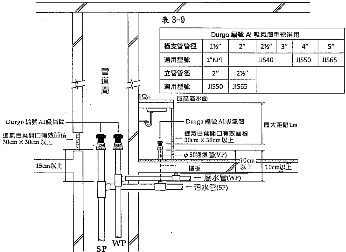
圖 3-12 污廢水伸頂通氣管、橫支管安裝 Durgo 編號 AI 吸氣閥圖示
