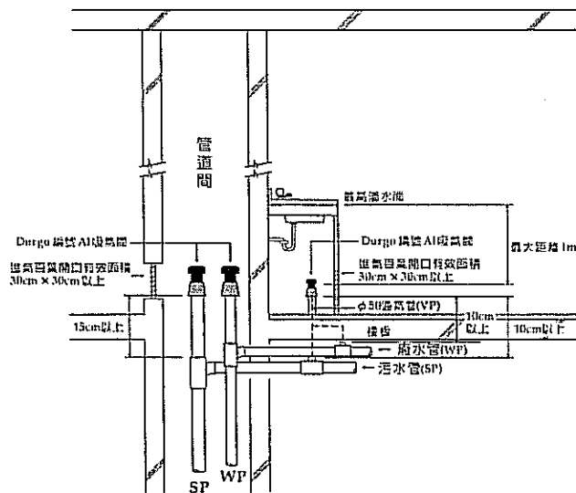
圖 2-4 污廢水伸頂通氣管、橫支管安裝 Durgo 編號 AI 吸氣閥圖
