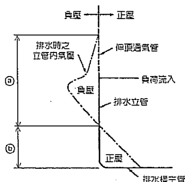
圖 3-1 排水通氣系統中伸頂通氣方式之排水管內壓力分佈
