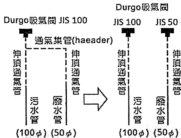
圖 3-4 伸頂通氣管需個別安裝 Durgo 吸氣閥圖示
