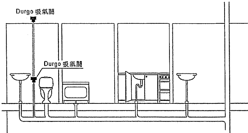
圖 3-3 排水橫支管安裝 Durgo 吸氣閥圖例
