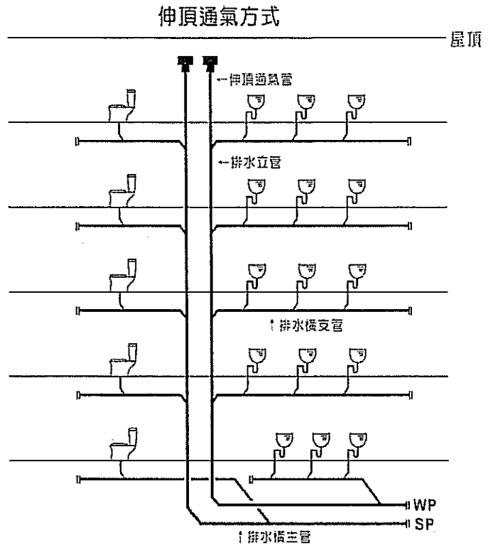
圖 3-5 伸頂通氣方式系統使用 Durgo 吸氣閥圖例
