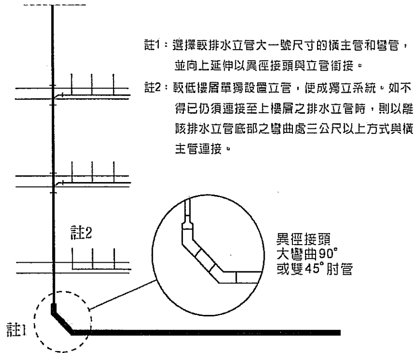
圖 3-11 排水立管底部及低樓層配管施工方式
