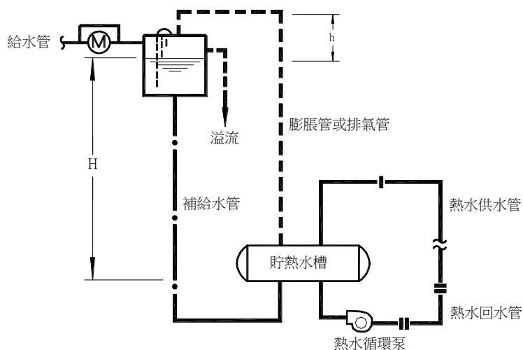
圖 A-10 熱水供給裝置之配管圖
