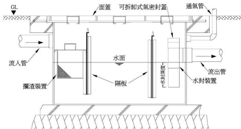
圖4-20 工廠製造的油脂截留器參考圖例
