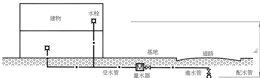
圖 A-3 自來水引入配管圖
