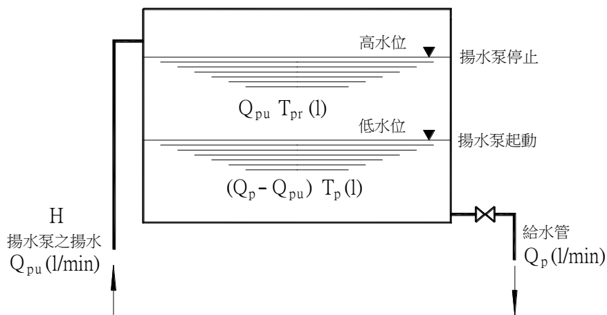
圖 A-1 高架水槽之容量
