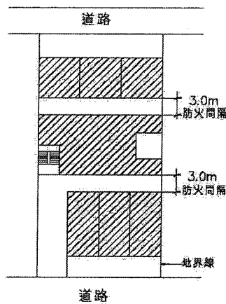
基地雖臨接二條道路，基地內因有兩種以上建築物，各處建築物之間仍應留設3m防火間隔。
