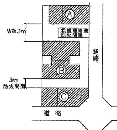
基地雖二面臨接二條道路，基地內各有兩種以上建築物，故各建築物間留設3m防火間隔，如圖中A、B、C之間，應留設3m防火間隔。
